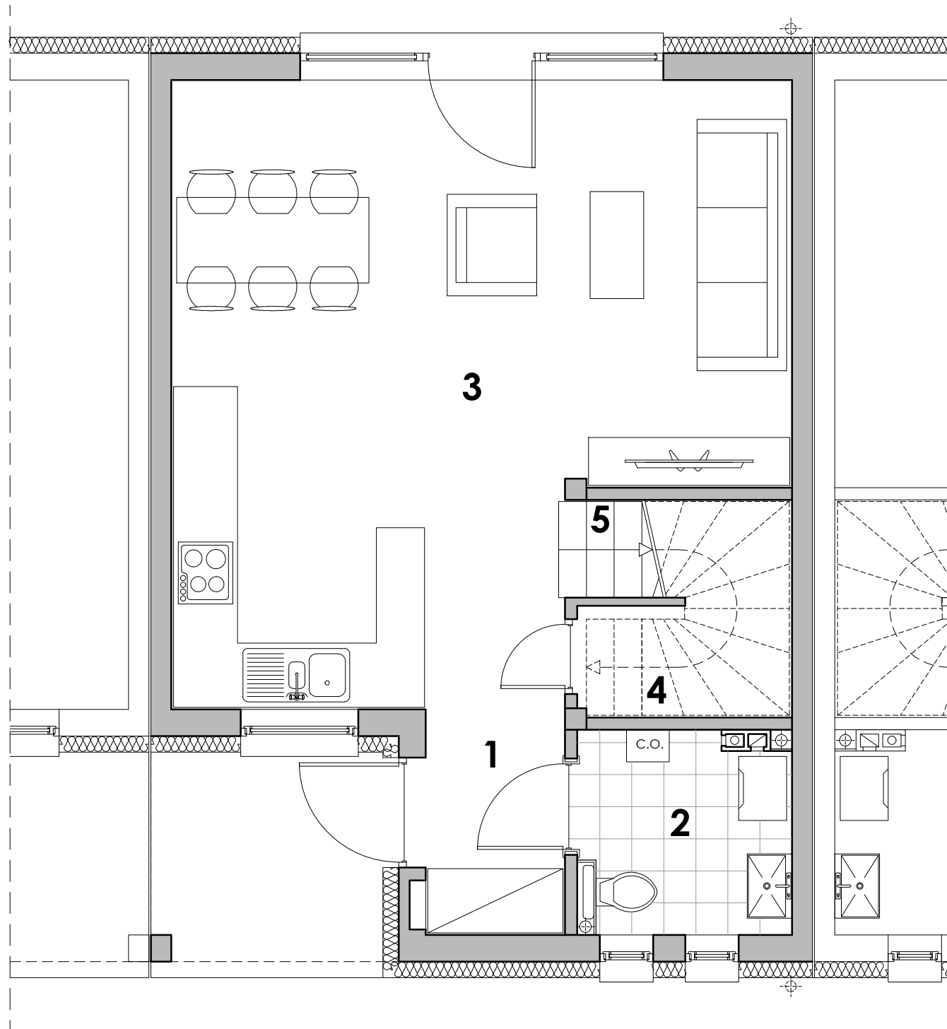
ZESTAWIENIE POMIESZCZEŃ parter
